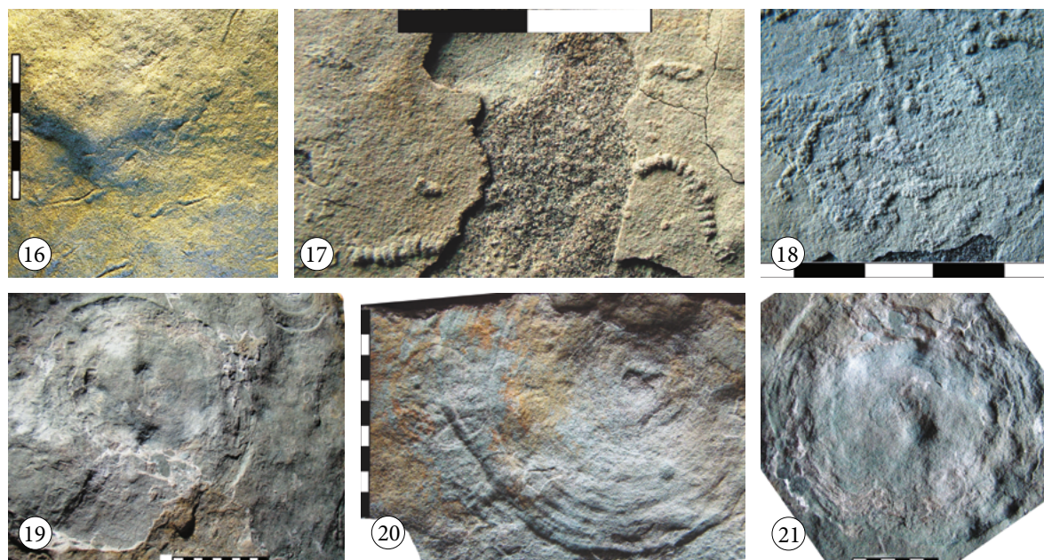
Fig. 16. Didymaulichnus nerodenkoi Grytsenko ichnosp. nov. Рис. 16. Didymaulichnus nerodenkoi Grytsenko ichnosp. nov.
